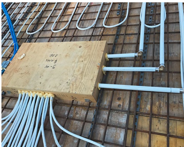
[FIG. 3] Exemple de caisson pour distributeur TABS.
